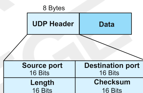
UDP Header
